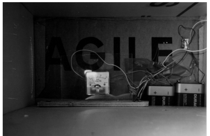
Photographie en vol d'un voltmètre relié à une thermistance placée à l'extérieur
